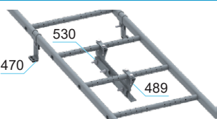
Konesaumakatto
